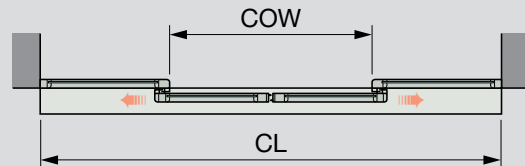
Двустворчатая дверь
